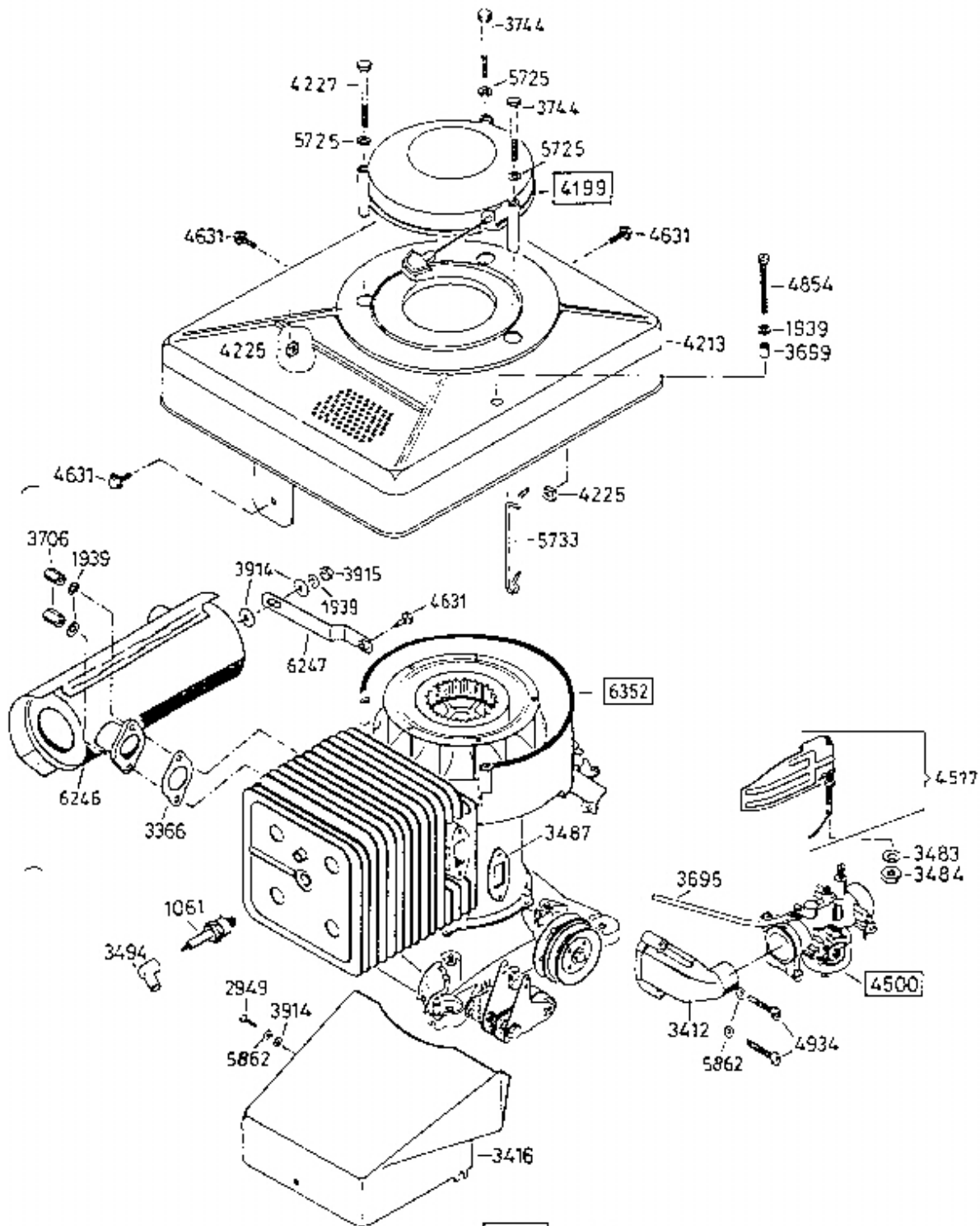
6351 Antriebsblock driving unit moteur complet
